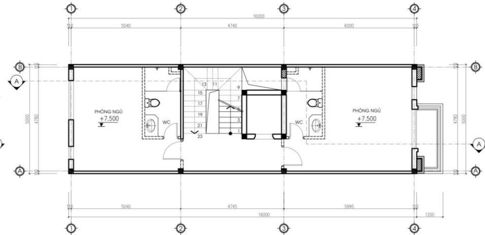
MẶT BẰNG TẦNG 3
