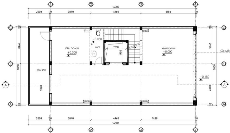
MẶT BẰNG TẦNG 1
