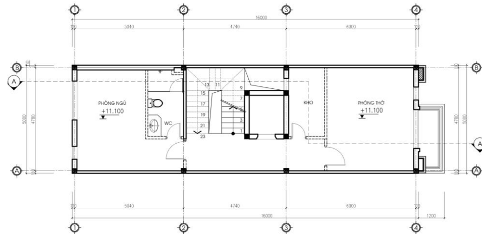
MẶT BẰNG TẦNG 4
