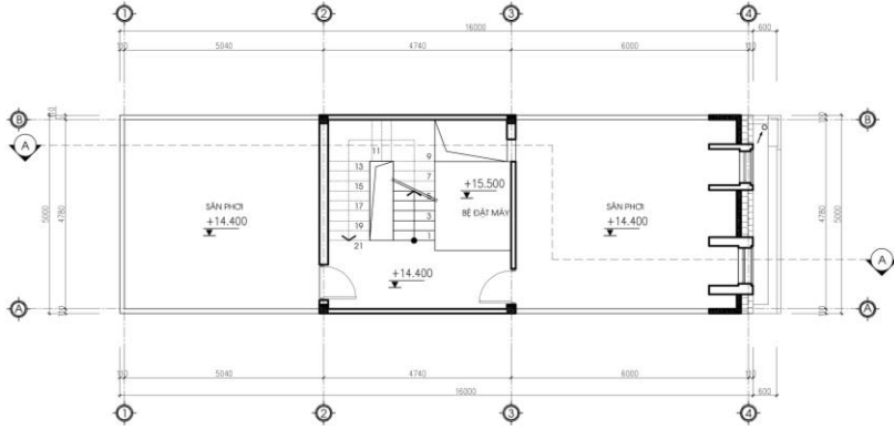
MẶT BẰNG TẦNG TUM
