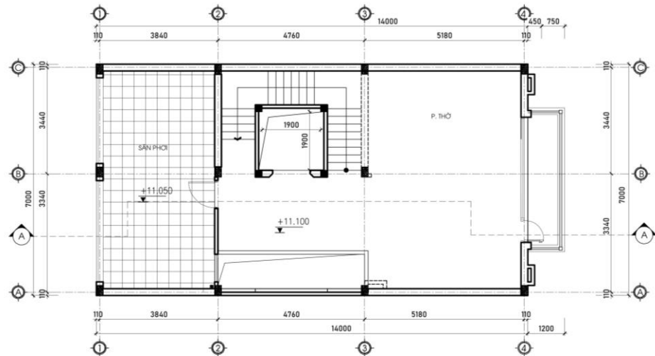
MẶT BẰNG TẦNG 4
