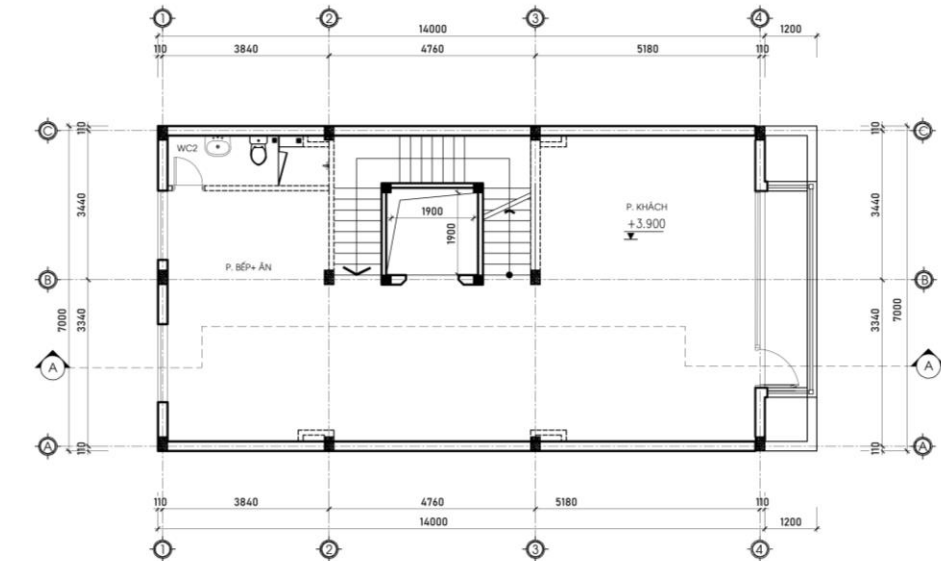
MẶT BẰNG TẦNG 2
