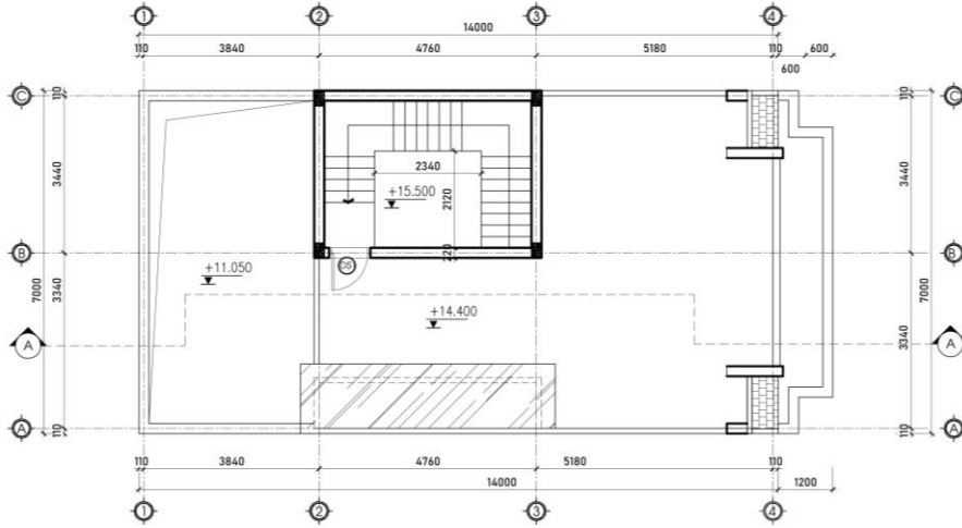
MẶT BẰNG TẦNG TUM
