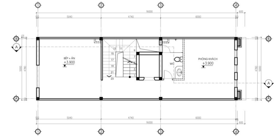
MẶT BẰNG TẦNG 2
