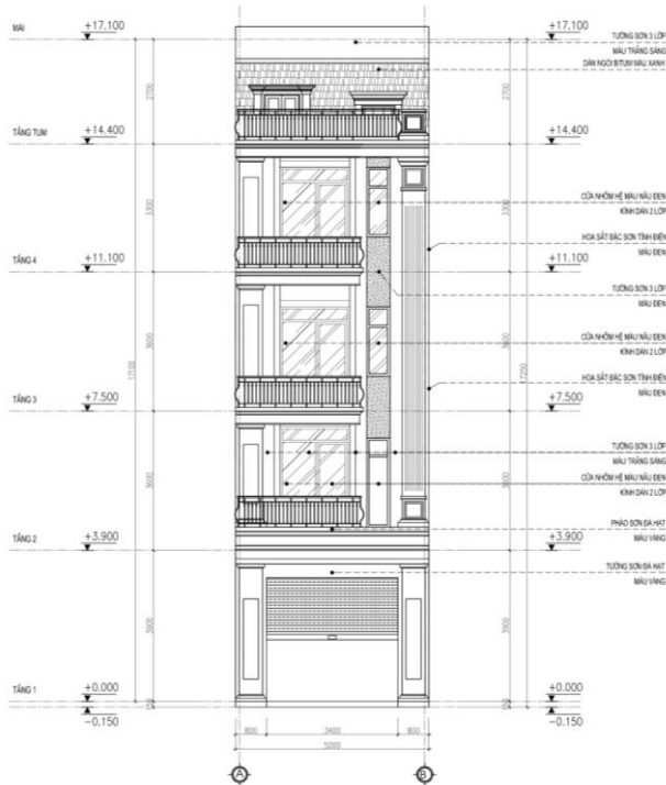
MẶT ĐỨNG TRỤC A-B
