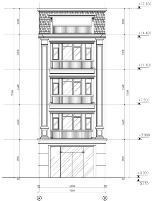
MẶT ĐỨNG TRỰC A-B
