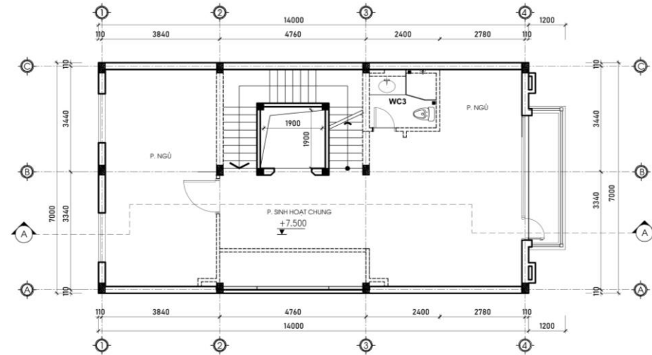
MẶT BẰNG TẦNG 3
