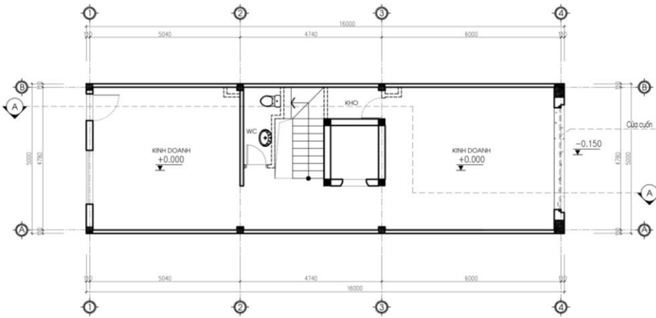
MẶT BẰNG TẦNG 1
